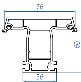
T-Mullion 2102-1101
