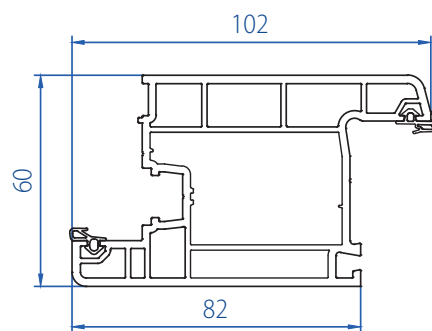
Inward Door Sash 2103-1104
