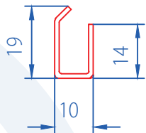
Eco Fly mesh Sash 1.5mm : 9405-1502
