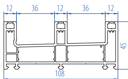
3T Sliding Frame 2104-3102
