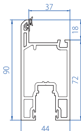
Sliding Door sash 3105-1103
