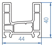
2T Frame 4104-3101
