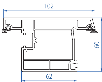
Outward Door Sash 2103-1102
