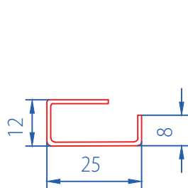
Frame 1.5mm :9501-1501
