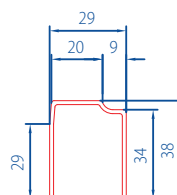
(Option-I) Sliding Sash 2mm:9205-2002
