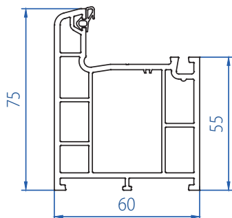
Door Frame 2101-1103
