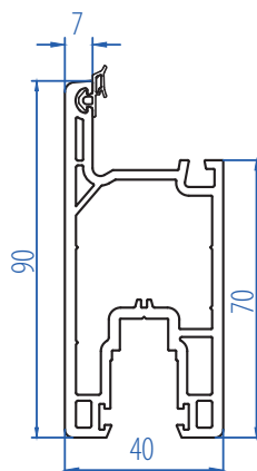
Sliding Door sash 2105-1103
