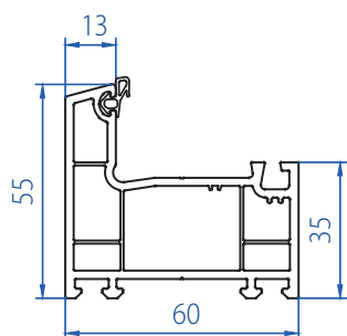
Casement Frame 2101-1101
