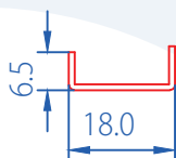
2T Frame 1.5mm : 9404-1501
