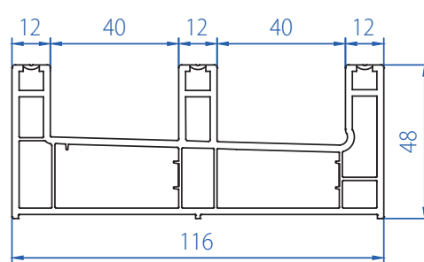
3T Sliding Frame 3104-3102
